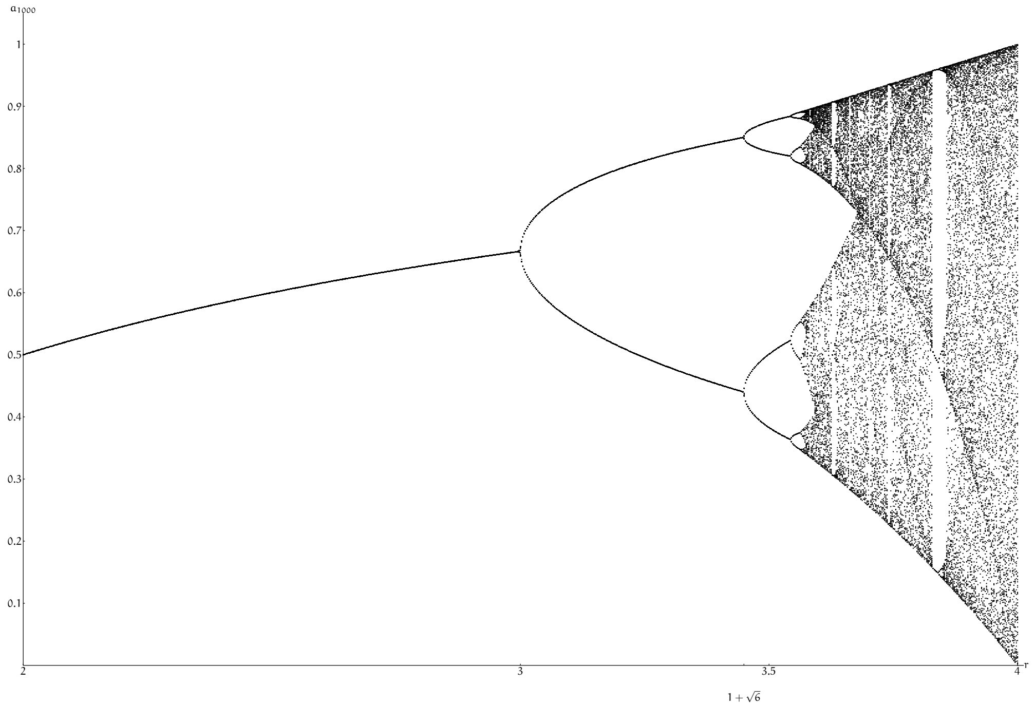
各 2 \leq r \leq 4 (横軸) に対して、様々な初期値 a_1 を取って a_{1000} の点をプロットしたグラフ
